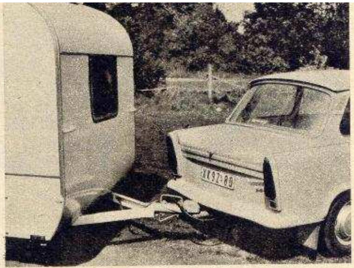
Bei kleinstem Wendekreis ist noch ausreichend Abstand zwischen Anhänger und Pkw.
