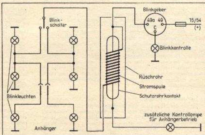
Schaltung und Aufbau des Stromrelais zur Funktionskontrolle bei Anschluß der Anhängerblinkleuchten an den Heckblinkleuchten des Pkw (Einkreisblinkanlage).
