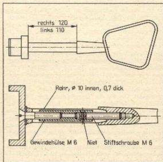
Die Verlängerungsrohre (rechts 125, links 115 mm lang) wurden entsprechend den Konusmaßen an den Spiegelteilen an einem Ende gestaucht und am anderen Ende aufgeweitet.
