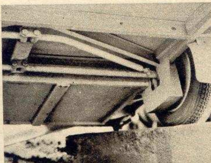
Die Räder des Wohnanhängers werden mit Pendelachsen geführt und mit Gummiblocken gefedert.
