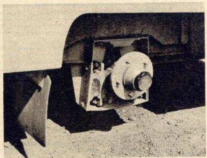
Die auf Schub beanspruchten Gummiblockfedern sind in Radnähe vor und hinter der Achse angeordnet.
